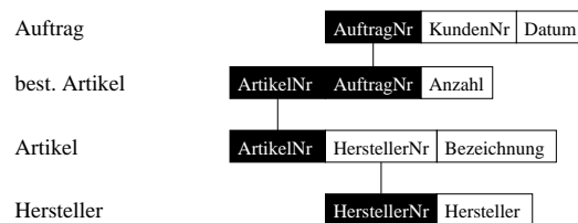
Abbildung 4.1: Streifendiagramm
