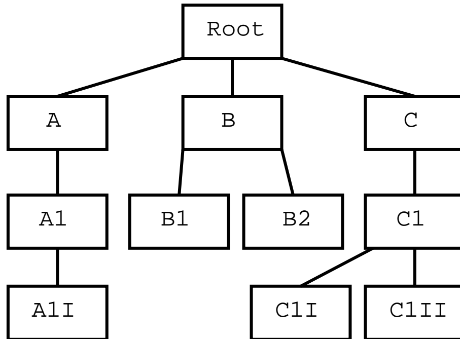
Abbildung 7.1: Unser Baum-Beispiel
