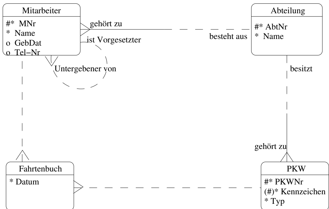
Abbildung 4.3: ER-Beispiel 2
